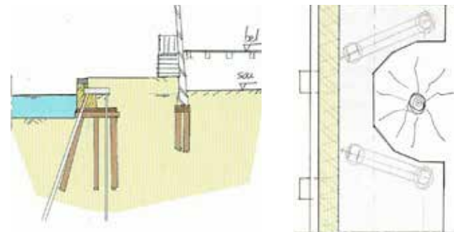
Versteviging bestaande constructie
